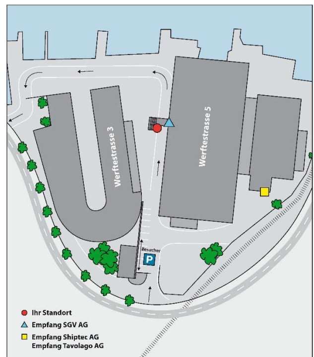
Situationsplanplan beim Treppenaufgang SGV 600x700mm
